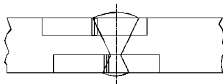
Lämpömuutosvyöhyke
