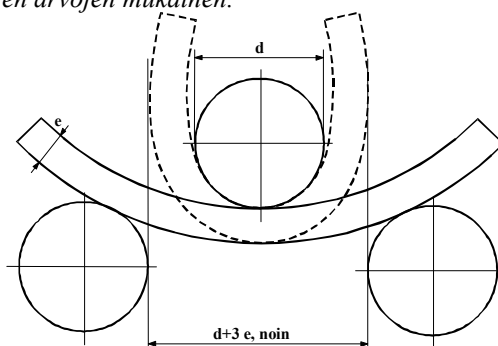
Taivutuskokeen kaaviokuva
